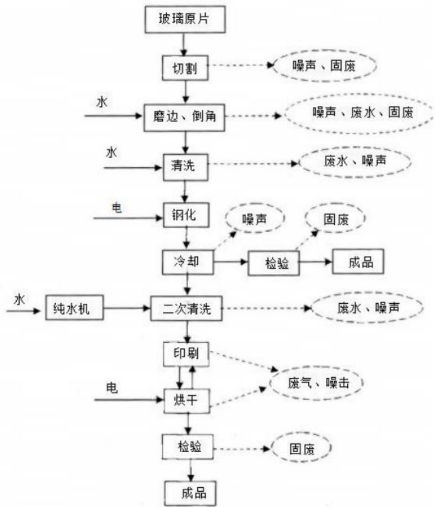
图 3-1 主要生产工艺流程图
